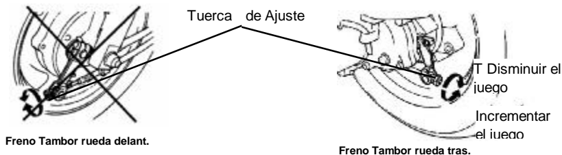
Freno Tambor rueda tras.
